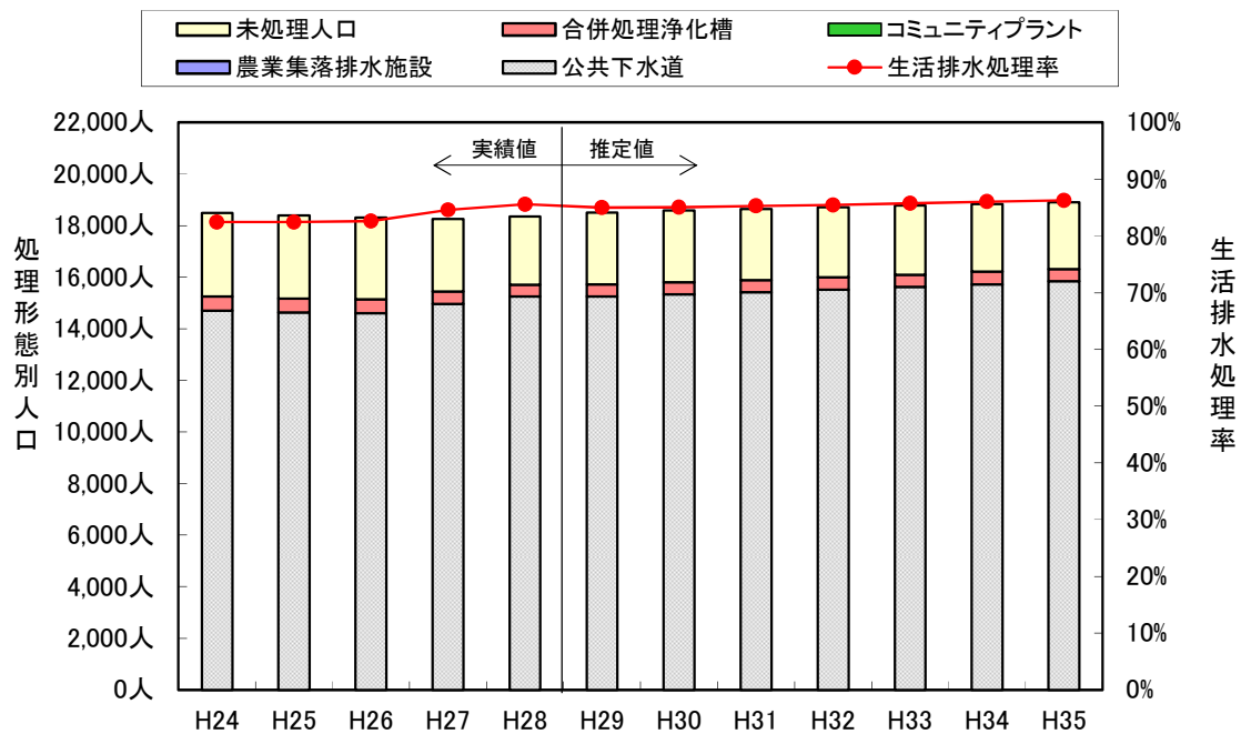
資料図-3 生活排水処理形態別人口トレンドグラフ（本業市）
